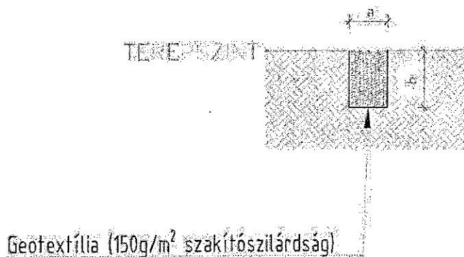
1. ábra- C-C' metszet, szikkasztó
