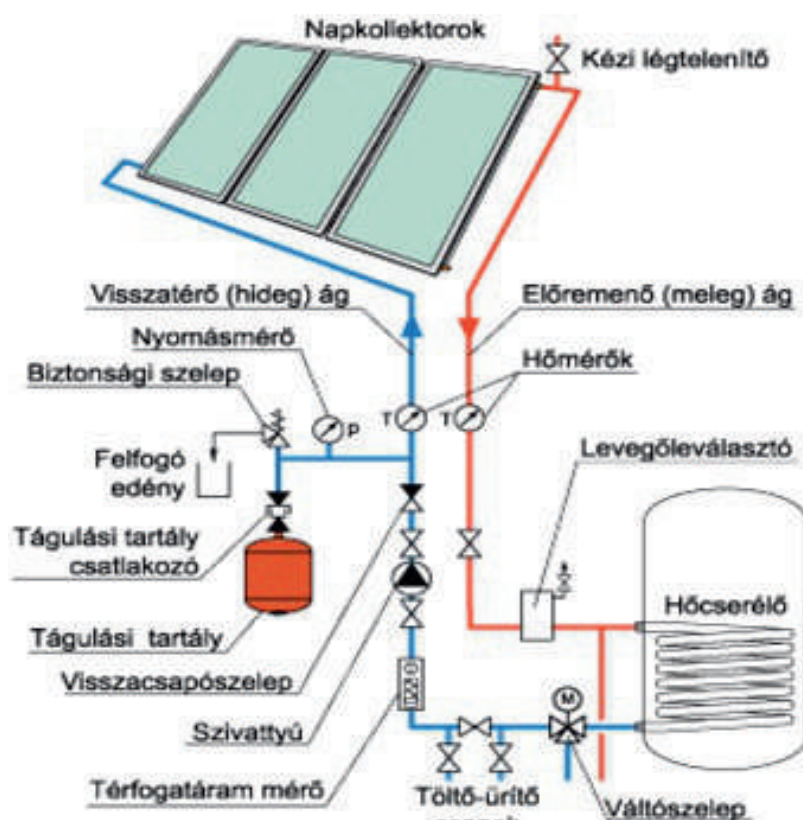
A napkollektoros rendszer működési modellje
