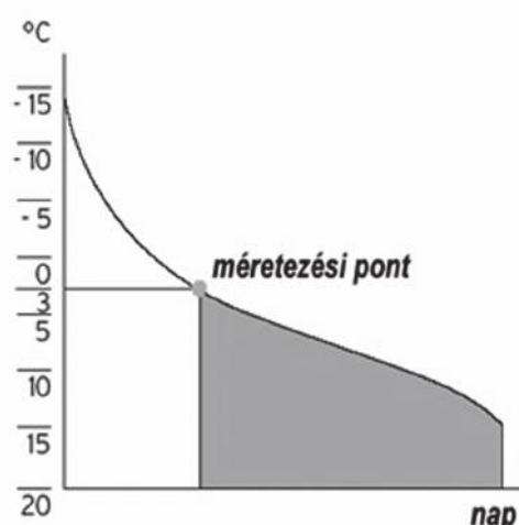
3. ábra Bivalens, alternatív üzemmód
