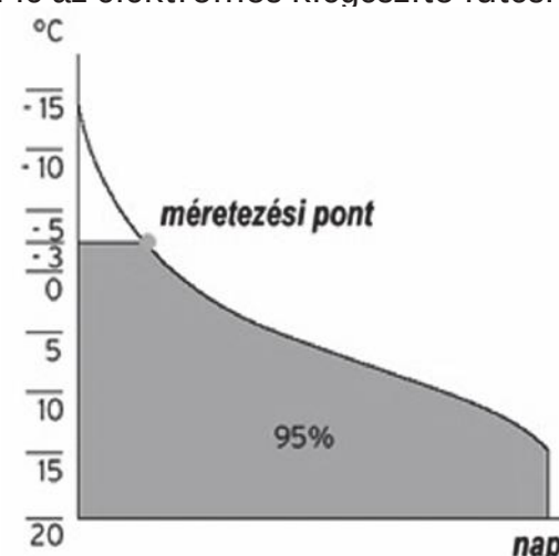
2. ábra Monoenergetikus üzemmód
