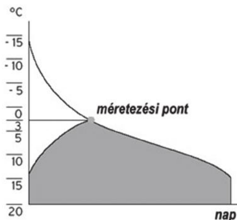
4. ábra Bivalens, párhuzamos üzemmód
