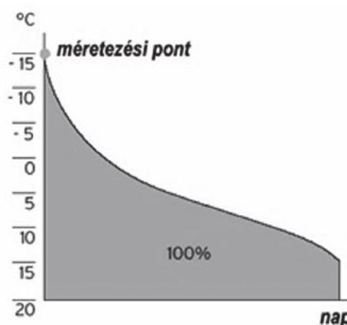
1. ábra Monovalens üzemmód
