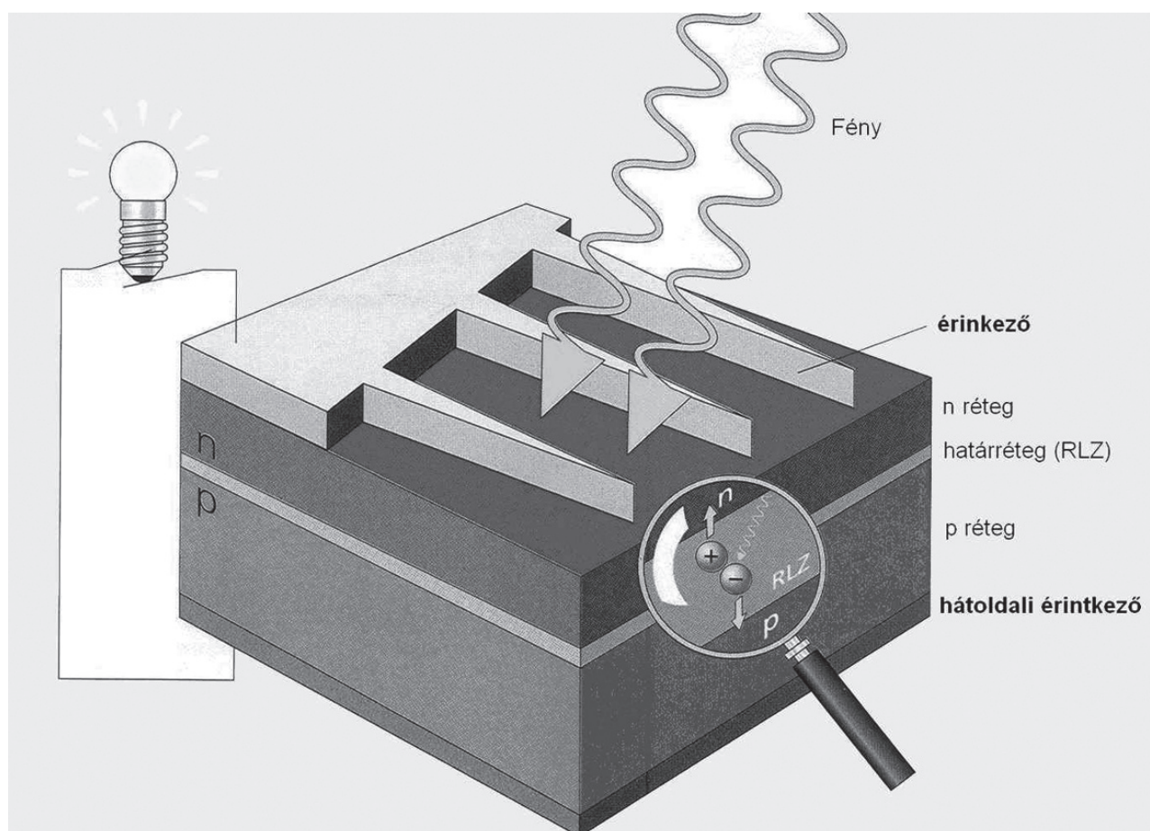
A napcella működési elve
