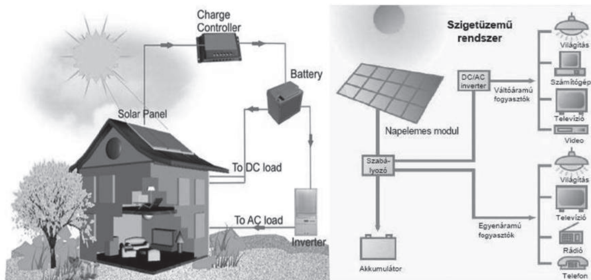
12 / 24 / 230 Voltos Sziget üzemű rendszer
