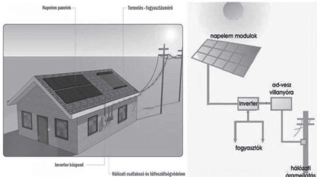
230 Voltos hálózatra kapcsolt rendszer
